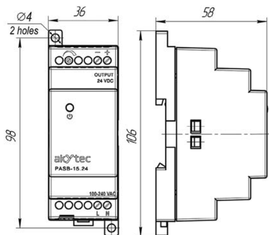
PASB-15.24
