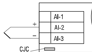
TC sensor wiring
