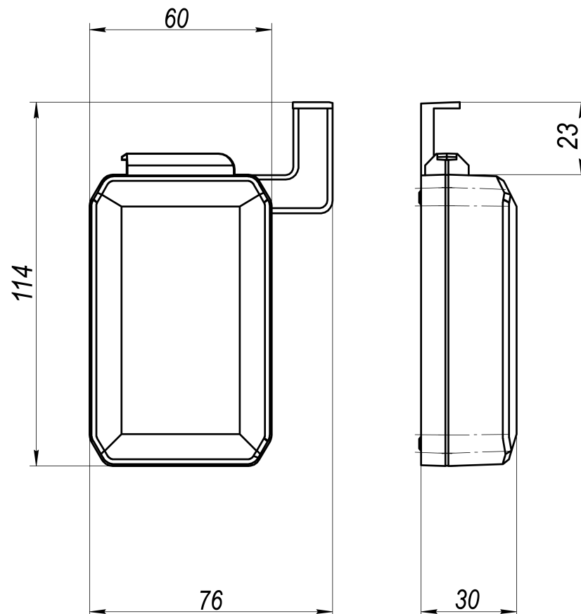
Abb. 2.1 Abmessungen
