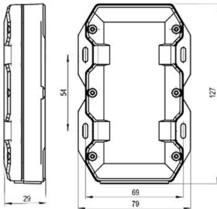
Fig. 2.1 Dimensions
