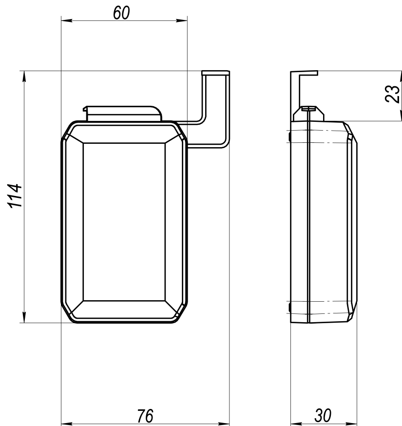
Fig. 2.1 Dimensions
