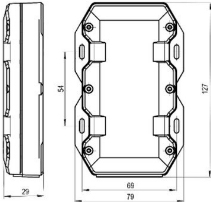
Abb. 2.1 Abmessungen
