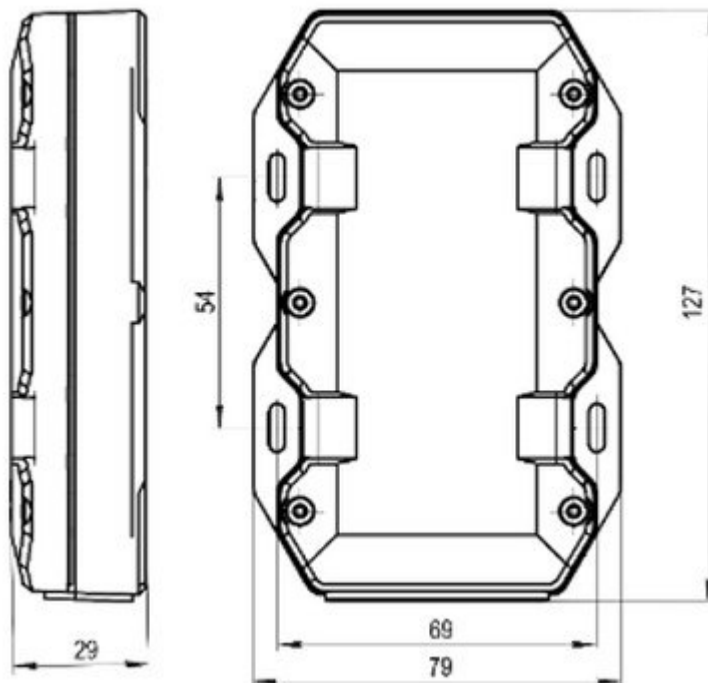
Abb. 2.1 Abmessungen
