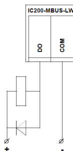
Abb. 8.3 Anschluss des externen Aktuators
