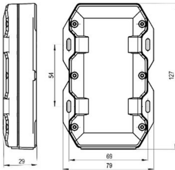
Abb. 2.1 Abmessungen
