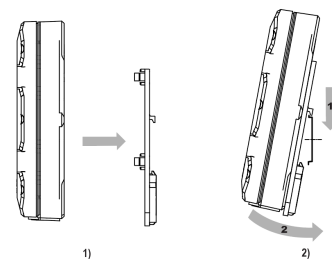
Abb. 6 DIN-Schienenmontage
