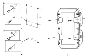
Abb. 7 Wandmontage
