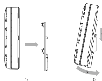
Fig. 6 – DIN rail mounting
