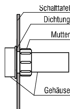
Abb. 5.4 Befestigung
