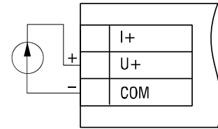
Fig. 5.6 Conexión sensor de Voltaje
