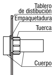
Fig. 5.4 Montaje
