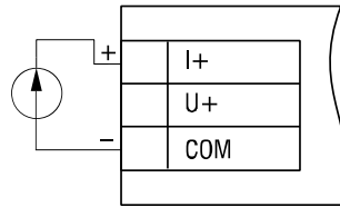
Fig. 5.5 Conexión sensor de corriente
