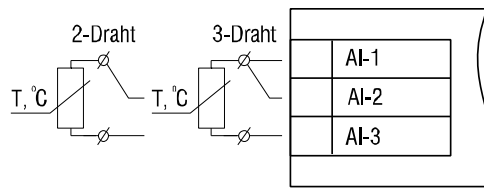
Abb. 5.5 RTD-Sensorverdrahtung
