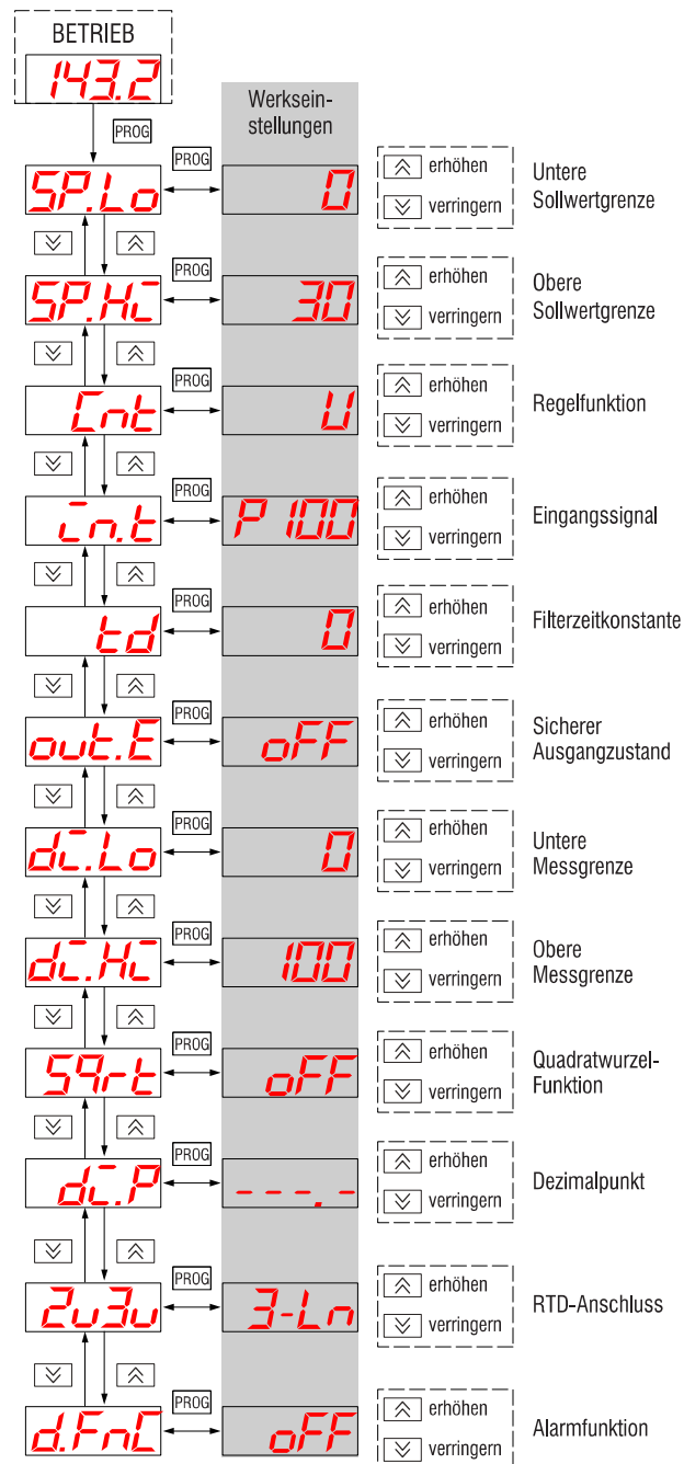
Abb. 7.1 Geräte-Menü
