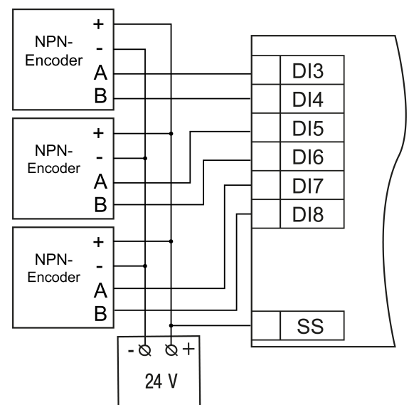
Abb. 5.8 Anschluss von AB-Encoder an NPN-Ausgänge
