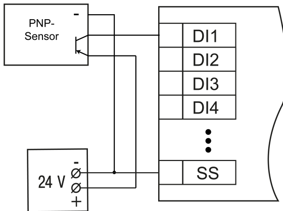
Abb. 5.5 Anschluss von 3-Draht-Sensoren an PNP-Ausgänge
