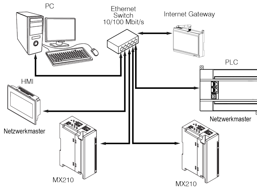
Abb. 5.10 Sterntopologie
