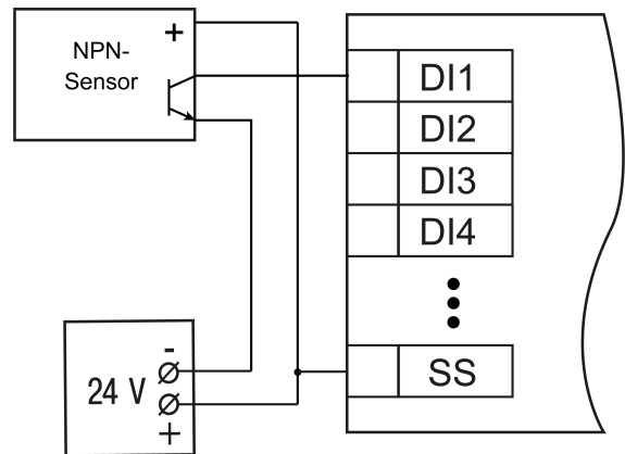
Abb. 5.6 Anschluss von 3-Draht-Sensoren an NPN-Ausgänge
