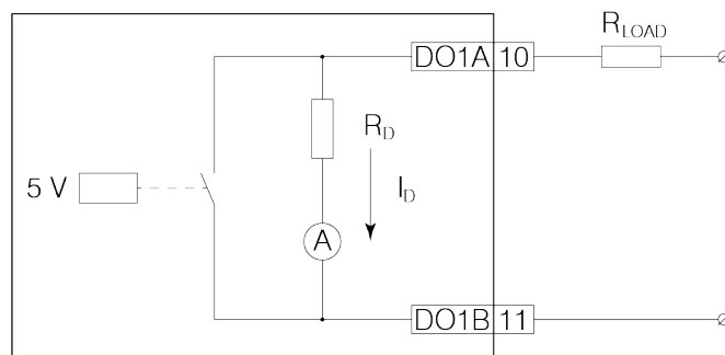
Abb. 4.2 Ausgangsdiagnose
