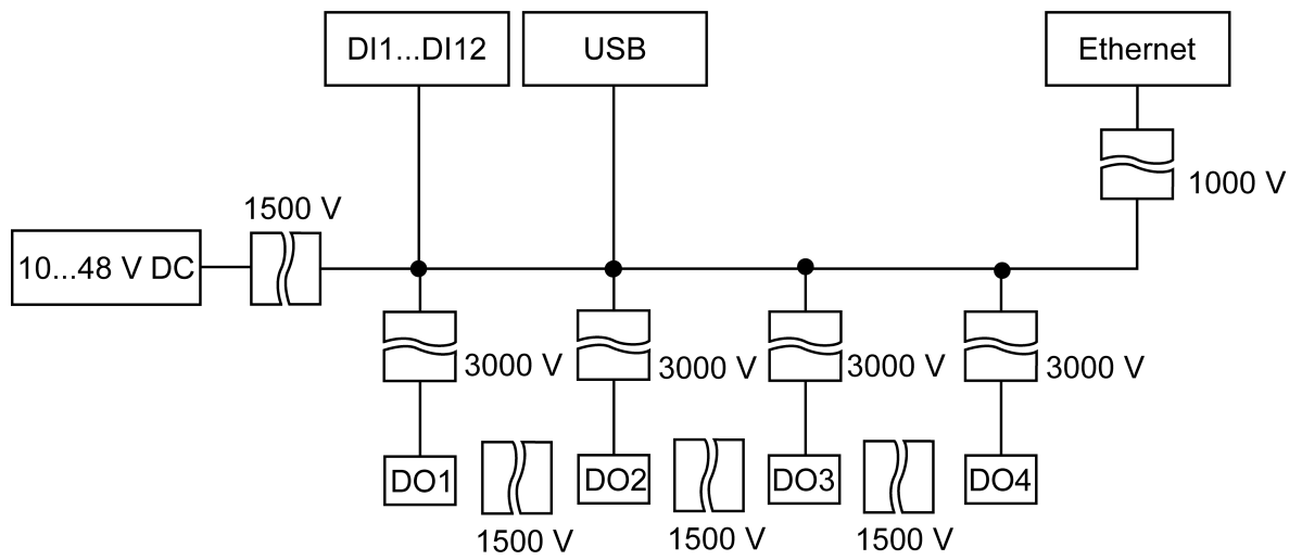
Abb. B.1 Isolierung der Gerätekomponenten
