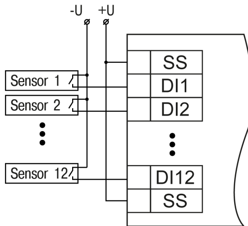
Abb. 5.4 Anschluss von Schaltkontakten
