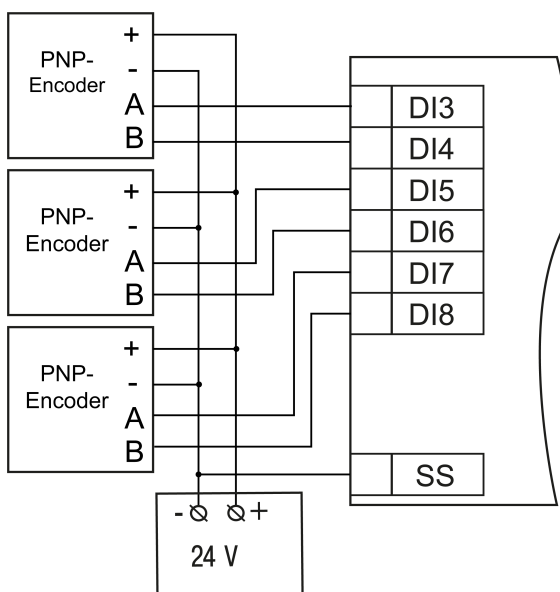
Abb. 5.7 Anschluss von AB-Encoder an PNP-Ausgänge
