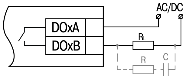
Abb. 5.9 Relaisausgänge
