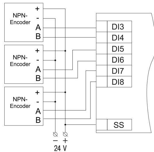
Abb. 5.11 Verdrahtung von NPN-Transistoren
