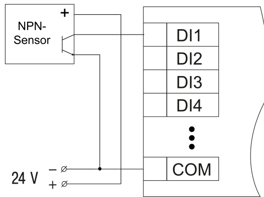
Abb. 5.9 Anschluss von NPN-Transistoren (nur für MV210-204)
