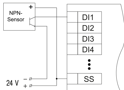
Abb. 5.8 Anschluss von NPN-Transistoren (nur für MV210-202)
