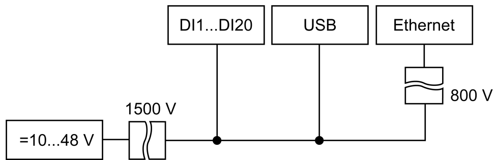
Abb. B.1 Galvanische Trennung
