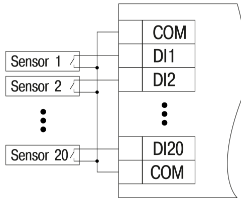
Abb. 5.6 Kontaktsensorverdrahtung (MV210-204)
