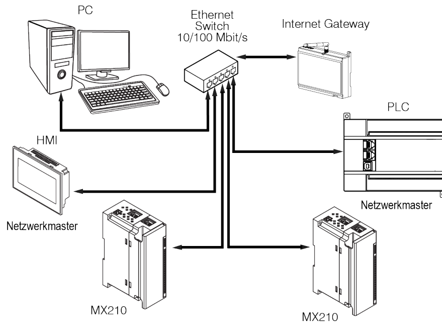
Abb. 5.12 Sterntopologie
