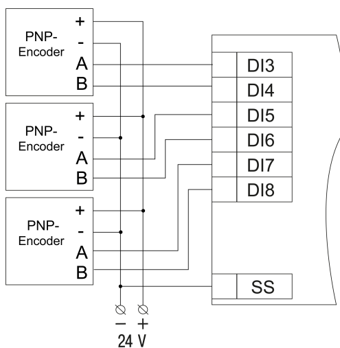
Abb. 5.10 Verdrahtung von PNP- Encodern
