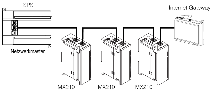
Abb. 5.13 Chain-Topologie
