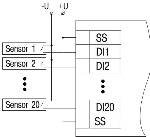
Abb. 5.4 Kontaktsensorverdrahtung (MV210-202) – Option 1
