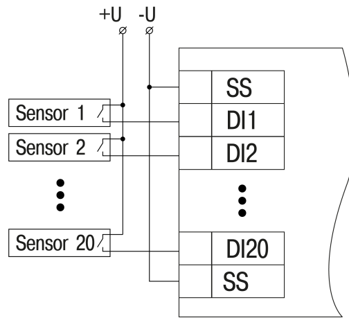
Abb. 5.5 Kontaktsensorverdrahtung (MV210-202) – Option 2
