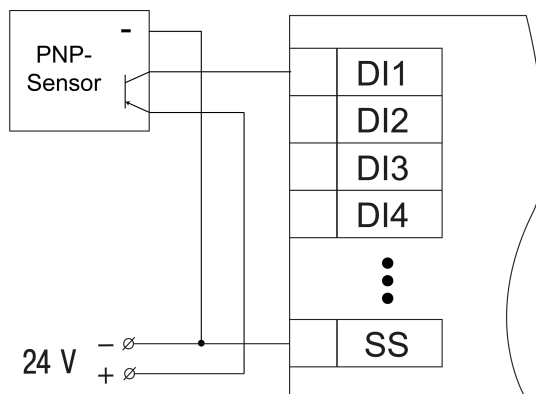
Abb. 5.7 Anschluss von PNP-Transistoren (nur für MV210-202)
