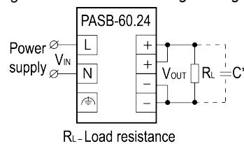
Fig. 7 – Wiring
