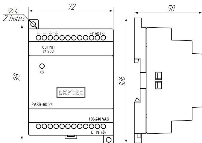
Fig. 5 – Dimensions
