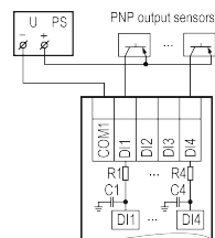
Fig. 3 – PNP transistor wiring
