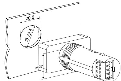
Abb. 5.3 Ausschnittmaße
