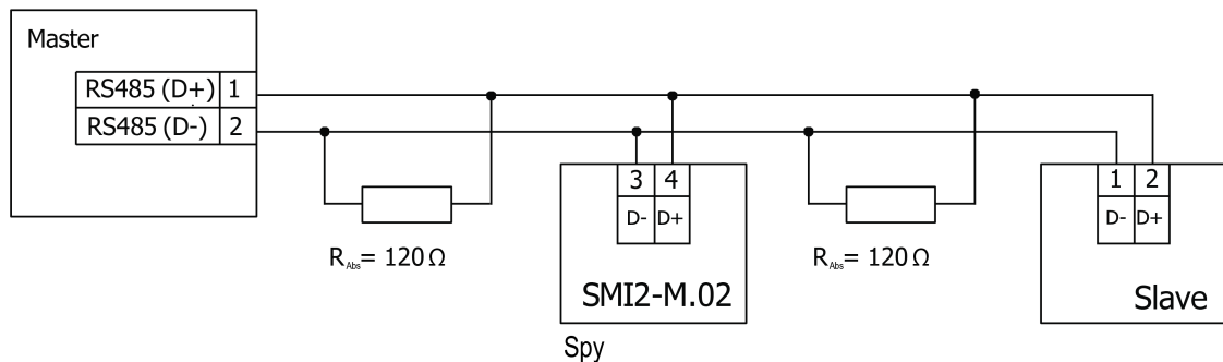
Abb. 5.6 SMI2-M.02 als Spy
