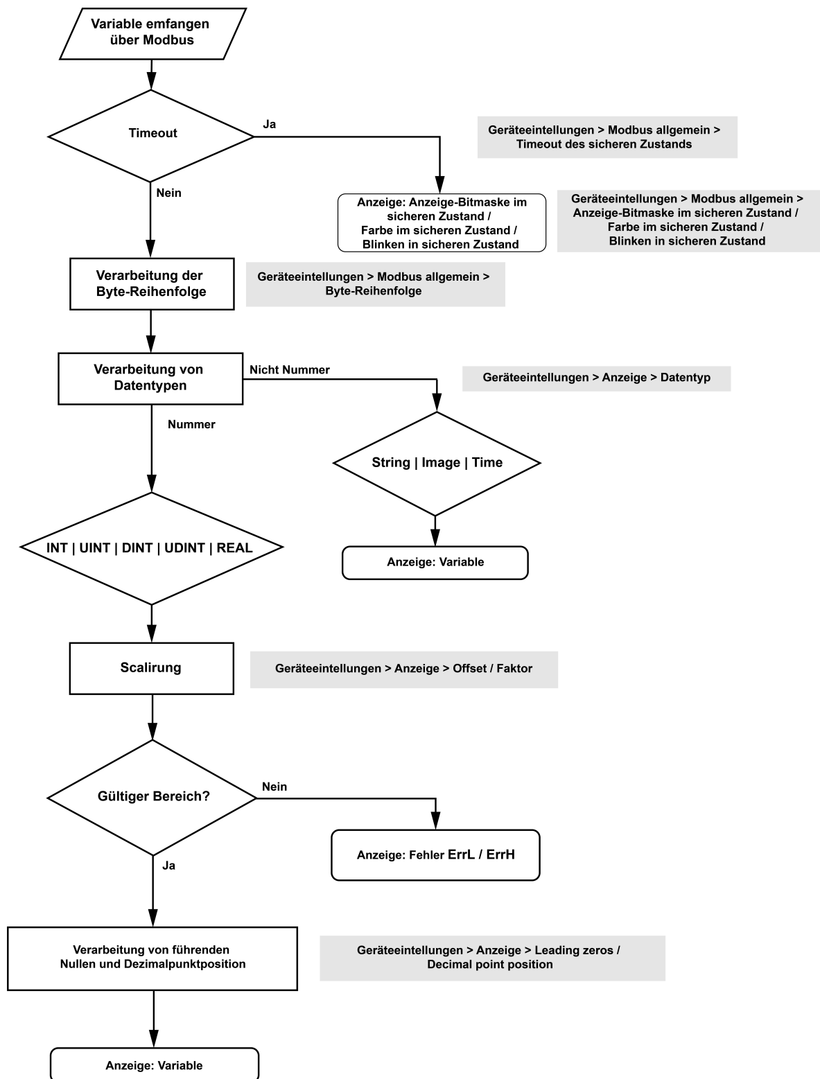
Abb. 4.1 Anzeige-Betriebsflussdiagramm
