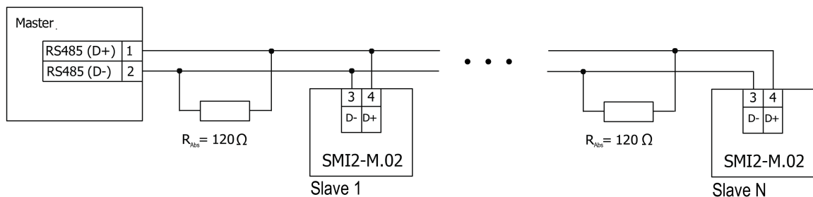
Abb. 5.5 Mehrere SMI2-M.02 als Slaves
