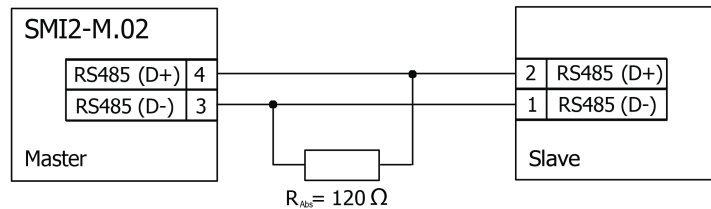
Abb. 5.4 Zwei SMI2-M.02 in Master-Slave-Verbindung
