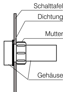
Abb. 5.2 Montage
