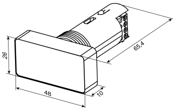
Abb. 5.1 Außenmaße
