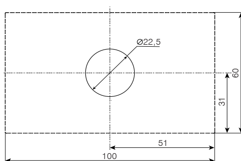
Abb. 4.2 Tafelausschnitte (Frontansicht)
